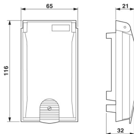
Dessin coté : VS-SI-EB-EMV-1
