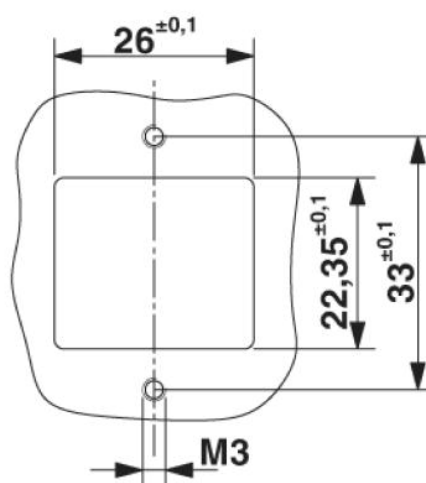
Découpe de montage
