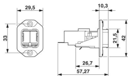
Cadre de montage Push-Pull SCRJ
