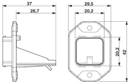
Cadre Push-Pull, système Freenet, IP67
