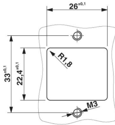
Découpe de montage
