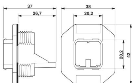
Cadre Push-Pull, système Freenet, IP67
