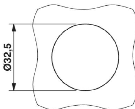
Découpe de montage
