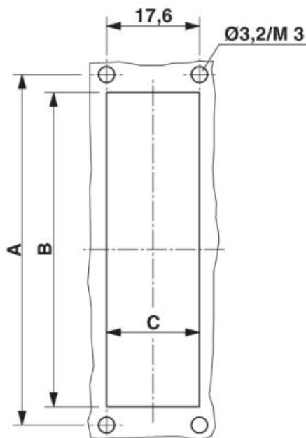
Découpe pour le montage : VS-25-A...
