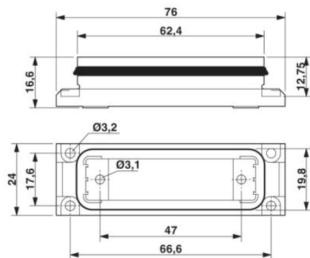
Cadre de montage SUB-D
