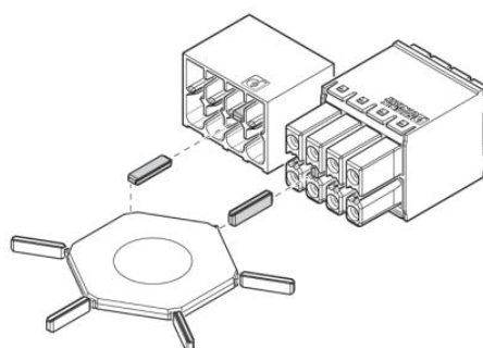
Utilisation de la languette de détrompage CP-DMC...
