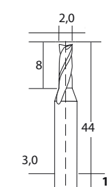
NO 28 761 Embouts de fraise à râper Pour la coupe et le fraisage de carreaux, de faïence, de bois et de plastique. Fraises de rechange pour FEX.
