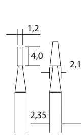
NO 28 752 Embouts de fraise à râper Pour la coupe et le fraisage de carreaux, de faïence, de bois et de plastique. Fraises de rechange pour FEX.
