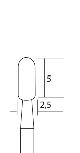
NO 28 272 Supports de rechange Axe 2,35 x 44 mm.
