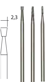
NO 28 758 Embouts de fraise à râper Pour la coupe et le fraisage de carreaux, de faïence, de bois et de plastique. Fraises de rechange pour FEX.
