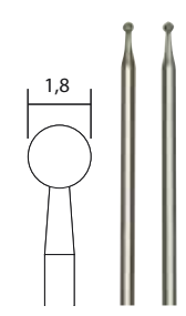
NO 28 222 Embouts de meulage diamantés Revêtement diamanté régulier. Profil de la tête et axe en acier inox. Pour le meulage, gravure et ciselage d'acier (aussi alliages au chrome-cobalt), de verre, de céramique, de porcelaine et de plastique. Axe \varnothing 2,35 mm.
