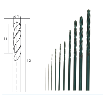
NO 28 874 Jeu de forets HSS DIN 338 \varnothing 0,3 – 0,5 – 0,8 – 1,0 – 1,2 – 1,5 – 2,0 – 2,5 – 3,0 – 3,2 mm. Pour métal non-ferreux, acier et acier inox. 10 pièces.
