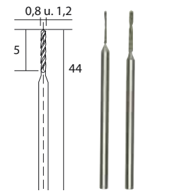
NO 28 255 Foret hélicoïdal diamanté pour forer des pierres semi-précieuses, etc. Axe \varnothing 2,35 mm.
