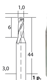
NO 28 759 Embouts de fraise à râper Pour la coupe et le fraisage de carreaux, de faïence, de bois et de plastique. Fraises de rechange pour FEX.
