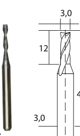
NO 28 760 Embouts de fraise à râper Pour la coupe et le fraisage de carreaux, de faïence, de bois et de plastique. Fraises de rechange pour FEX.
