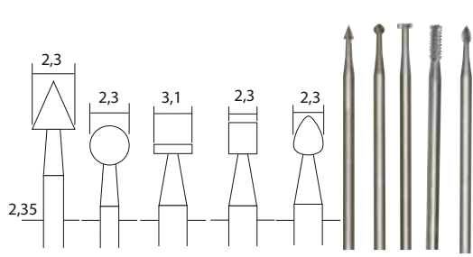
NO 28 710 Usure précise, concentricité parfaite et élasticité constante. Ils sont idéaux pour travailler, former, profiler et rainurer. Pour le
