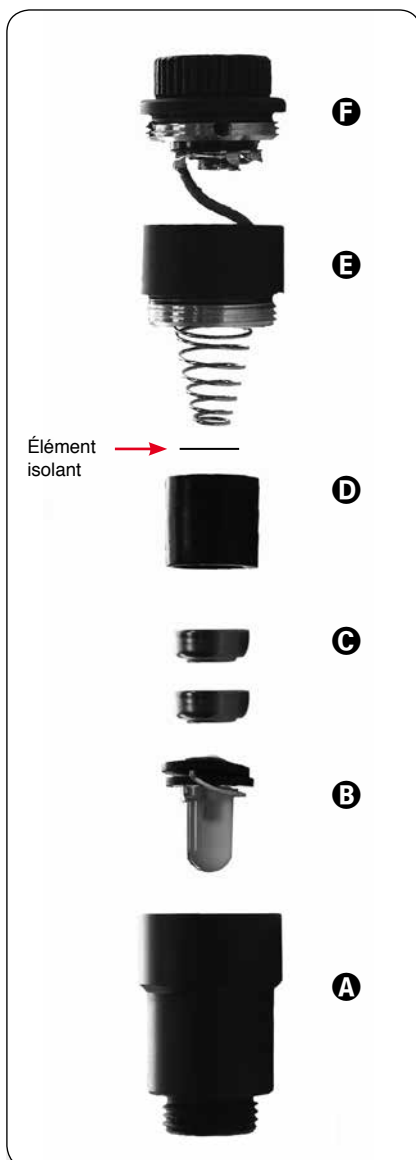
* Fig. 13a: éclairage du réticule: (A) Compartiment du réticule (B) Diode (C) Piles (D) Porte piles (E) Capot (F) Commutateur „Marche/Arrêt“
