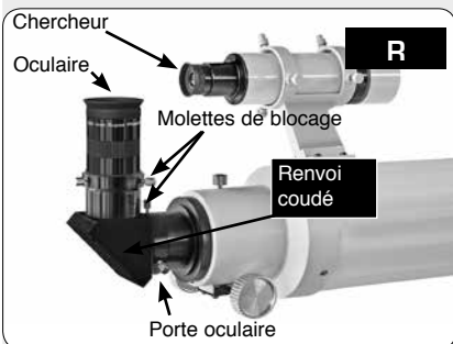
Fig. 10b: insertion du renvoi coudé et de l'oculaire dans le porte oculaire de la lunette
