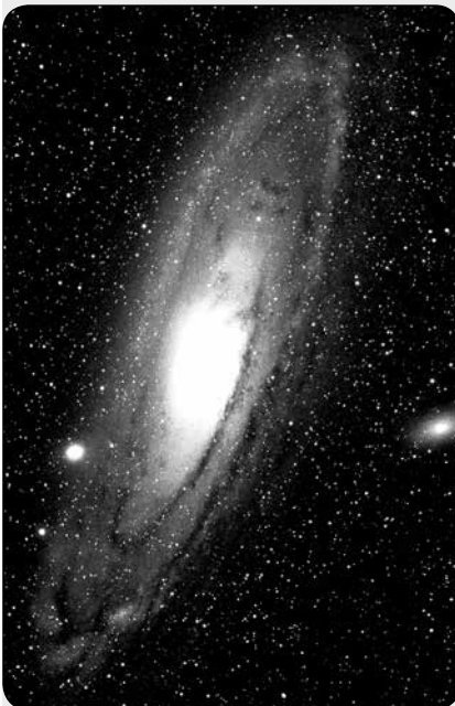
Fig. 29: la galaxie M31
