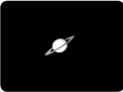
Fig. 25: Saturne avec son système d'anneaux.
