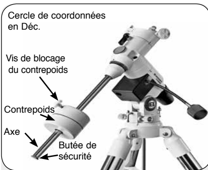
Fig. 6: Fixation du contrepois (cas de la monture EXOS 2)
