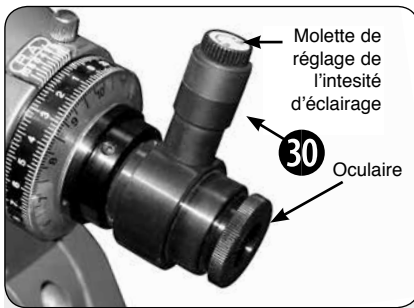
Fig. 19: le viseur polaire*
