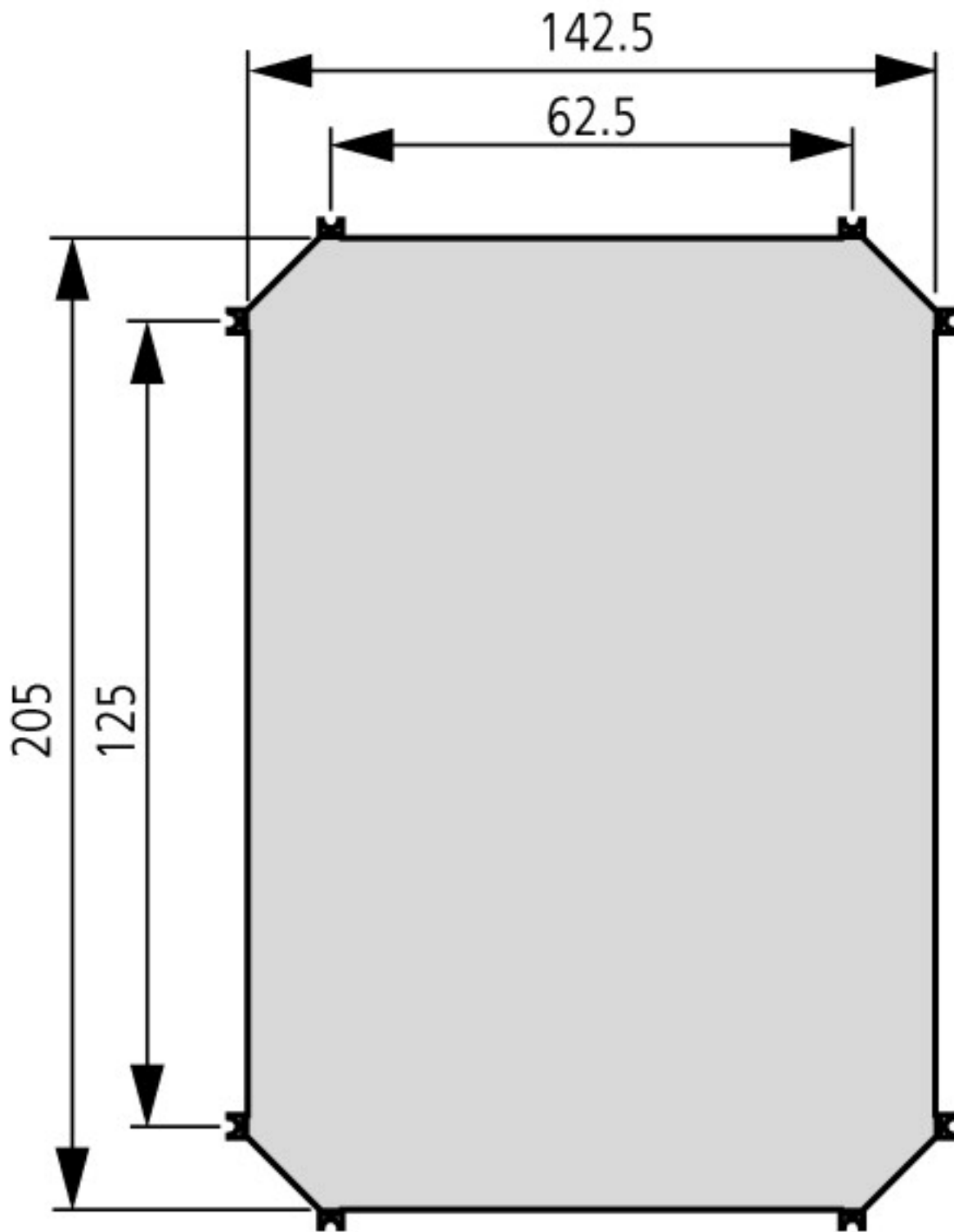
Platine de montage M3-... : 3 mm d'épaisseur
