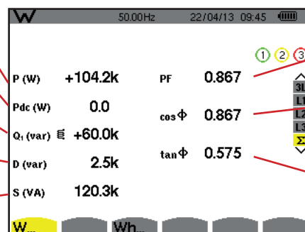
Figure 115 : l'écran d'affichage des puissances et des grandeurs associées totales en \Sigma
