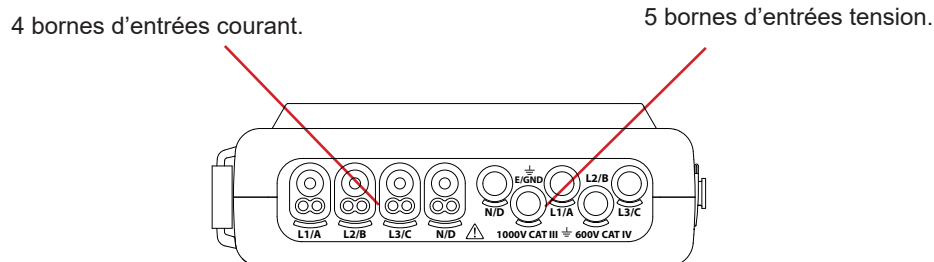
Figure 3 : les bornes de branchement
