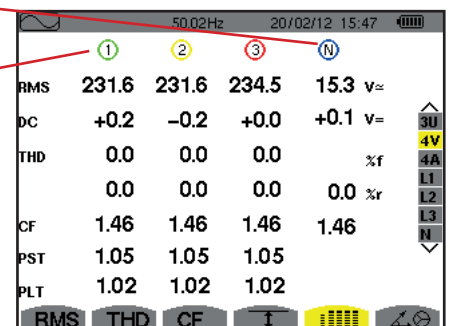
Figure 79 : l'écran affichage simultané en 4V
