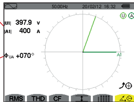
Figure 84 : l'écran d'affichage du diagramme de Fresnel en Diphase 2 fils
