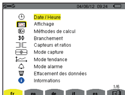
Figure 8 : l'écran Configuration
