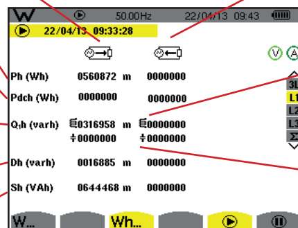
Figure 114 : l'écran d'affichage énergies consommées et générées en L1
