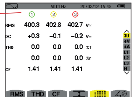
Figure 78 : l'écran affichage simultané en 3U
