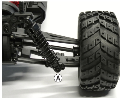
Bild 8: Hinterachse
