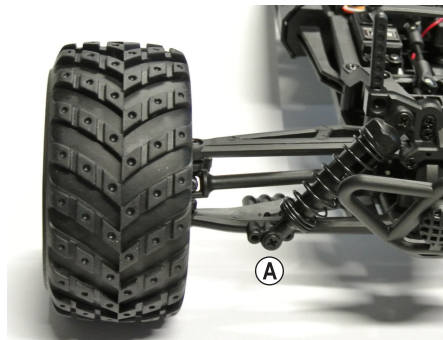
Bild 7: Vorderachse
