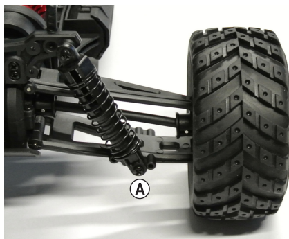
Afbeelding 8: Achteras
