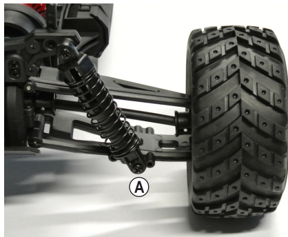
Figure 8 : Essieu arrière
