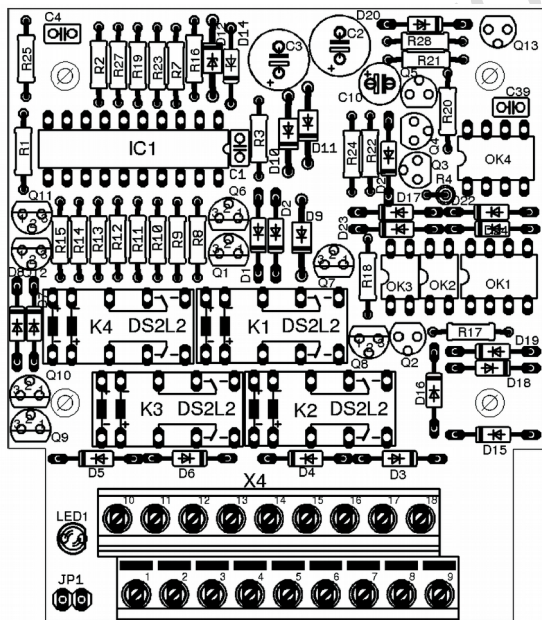
Fig. 1 : Plan d'implantation (SD-34)
