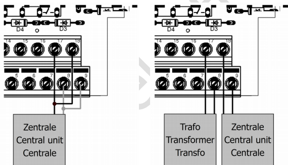
Fig. 2: Alimentation par la centrale
