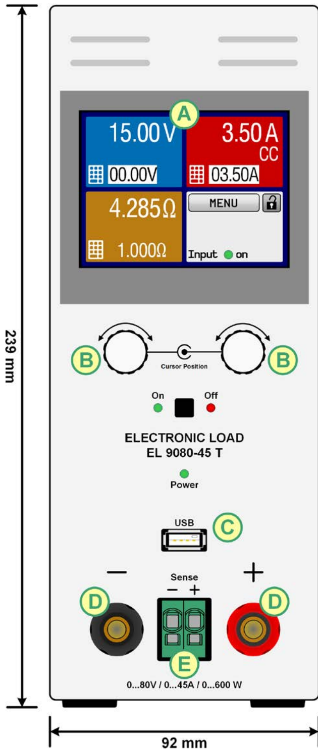
Figure 1 - Face avant
