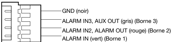
Caractéristiques de câble d'alarme 4P (accessoire)
