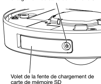
Vis de fixation de volet de fente de chargement de carte de mémoire SD
