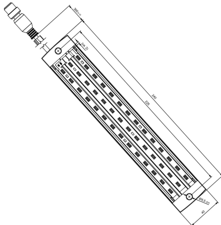
Dessin coté
