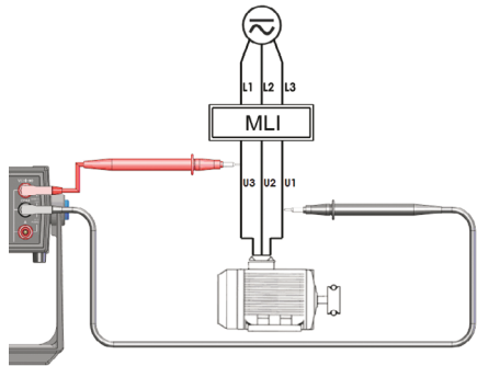
Exemple : mesure de tension sur un variateur
