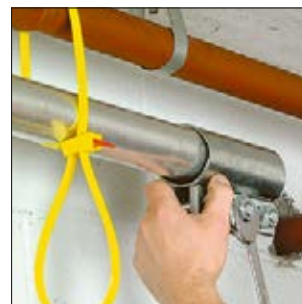
Le collier SpeedyTie convient aux applications temporaires et fait office de 3 ème main pour l'installateur.
