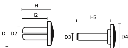
Composant 1 - Rivet TY8P2, constitué de 2 pièces
