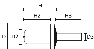
Rivets TY3P1 et TY8P1
