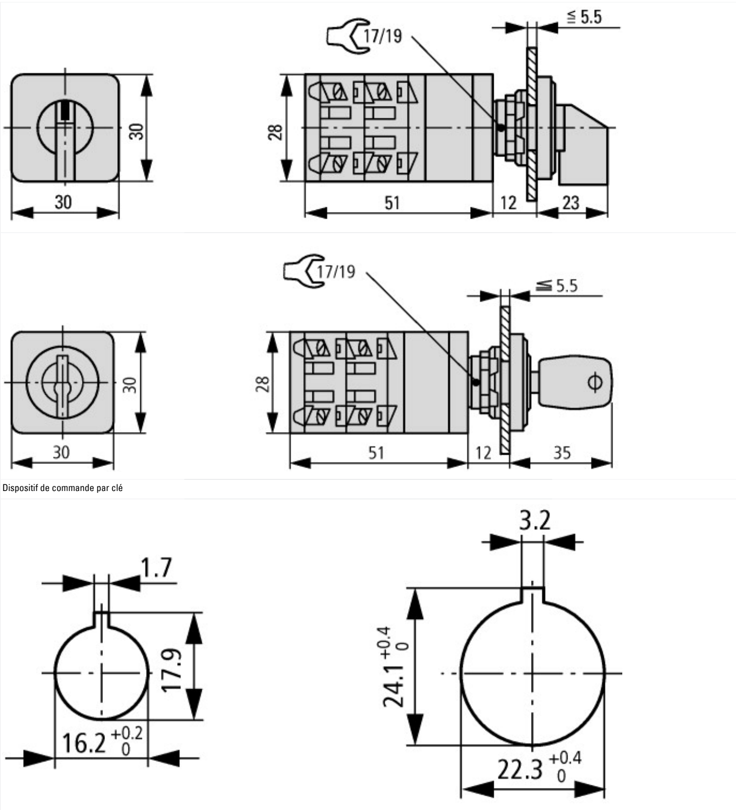
Dimensions de perçages, porte Dimensions de perçage au choix : 16,2 mm = sans réduction \triangle RMQ16 ; 22,3 mm = avec réduction \triangle RMQ Titan
