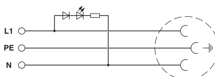
Schéma de connexion
