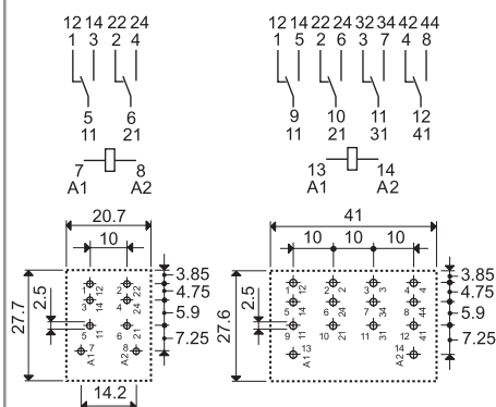
56.42 Vue coté cuivre
