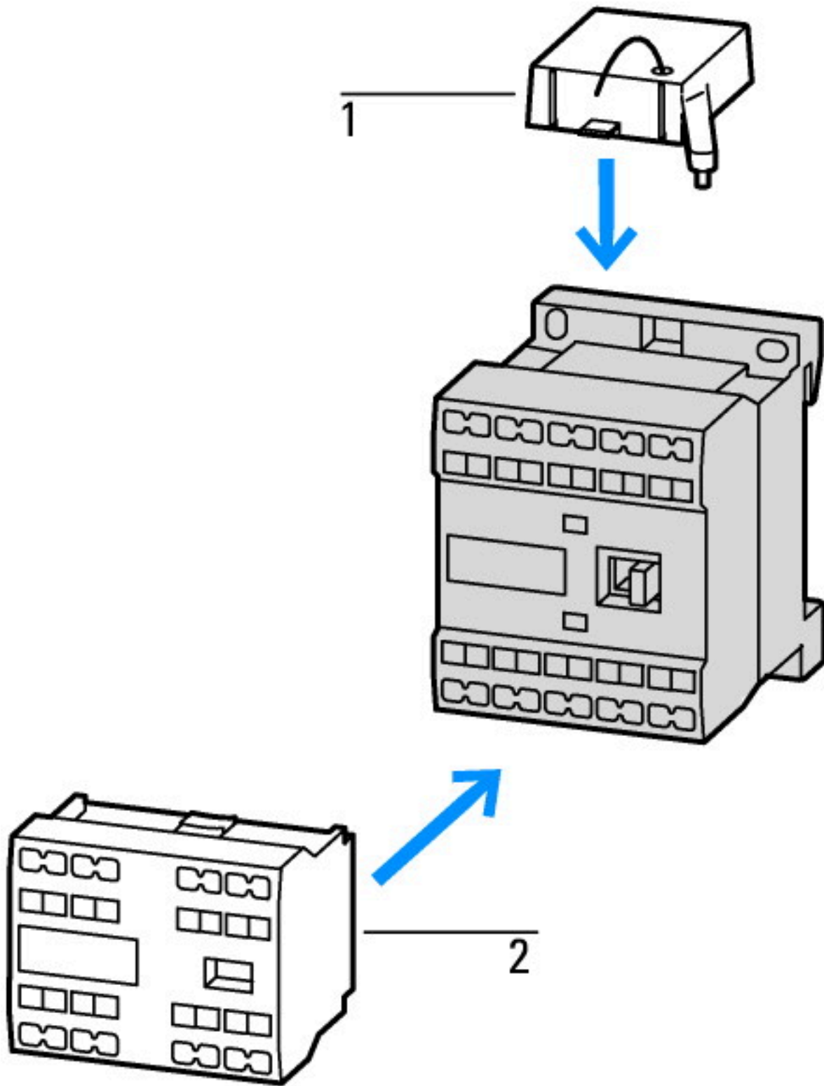
1 : Module de protection 2 : Modules de contacts auxiliaires Enveloppe entièrement isolée
