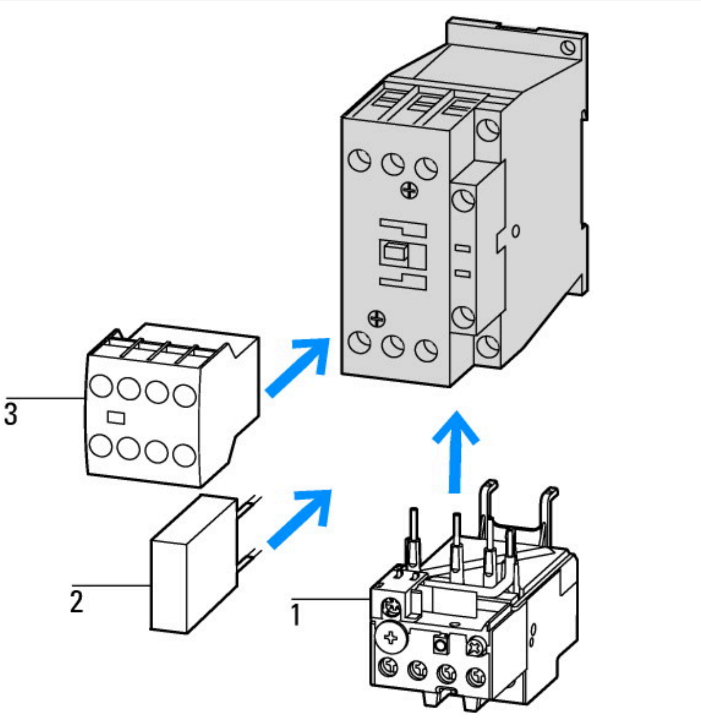
1 : Relais thermiques
