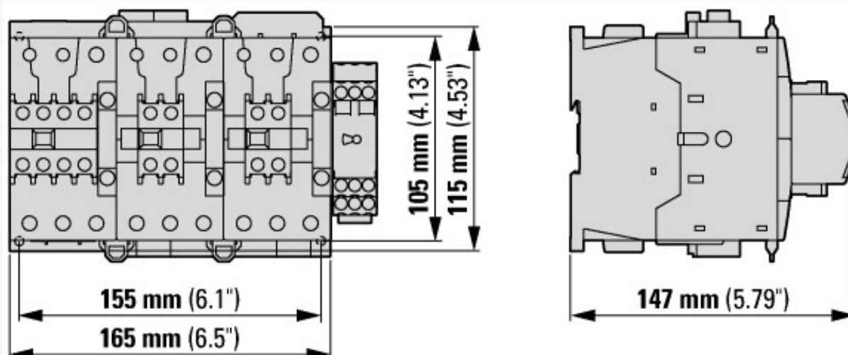
Appareil de base avec module de contacts auxiliaires
