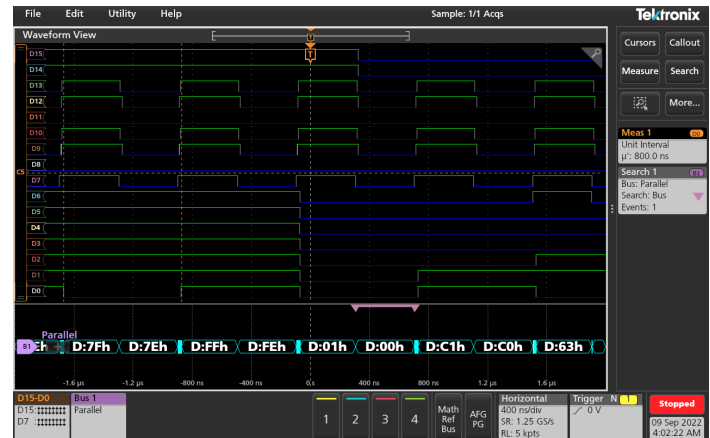
Déclenchement et décodage de voies numériques
