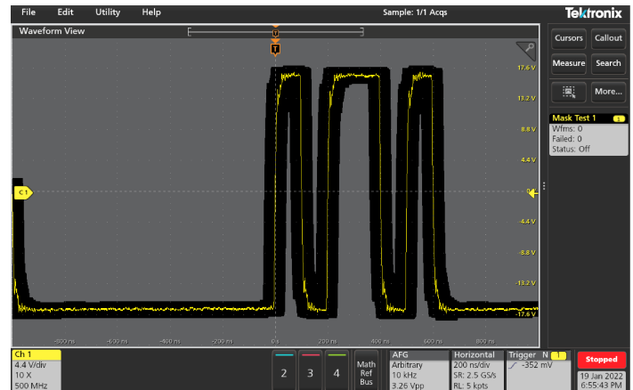
Test de limite de masque basé sur le signal de référence idéal
