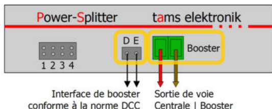
Face avant du Power-Splitter Version "Appareil fini"
