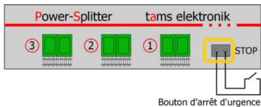
Face arrière du Power-Splitter Version "Appareil fini"
