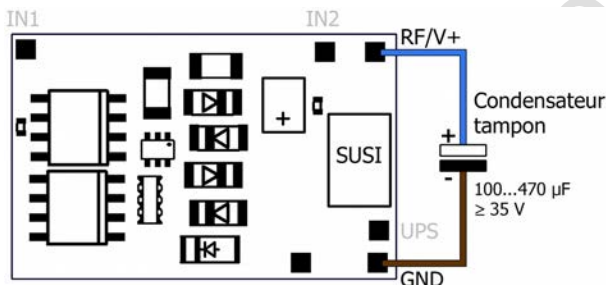
Raccordement d'un condensateur de soutien
