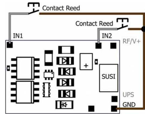
Raccordement de contacts Reed aux entrées de commutation
