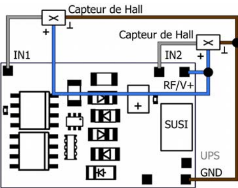
Raccordement de capteurs à effet Hall aux entrées de commutation
