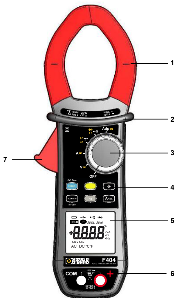
Figure 1 : la pince multimètre F404
