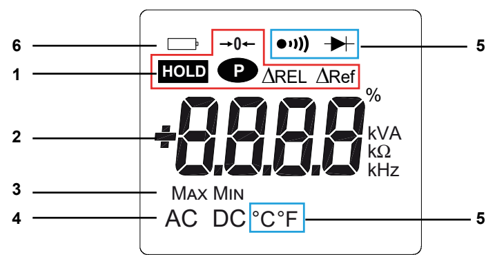
Figure 4 : L’afficheur
