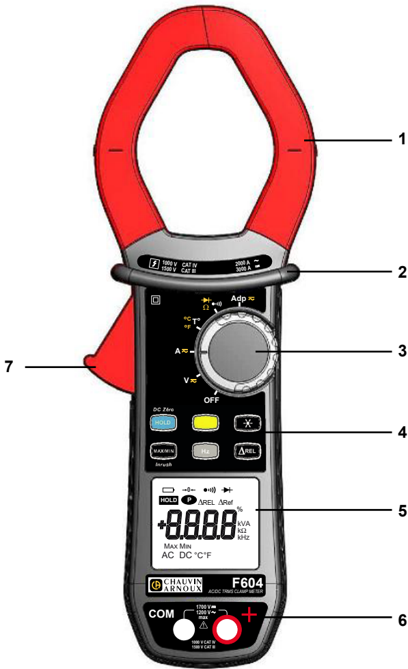
Figure 1 : la pince multimètre F604
