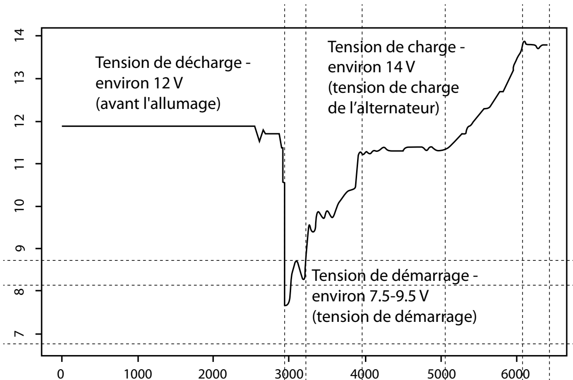
Analyse de la tension d'un véhicule lors d'un démarrage
