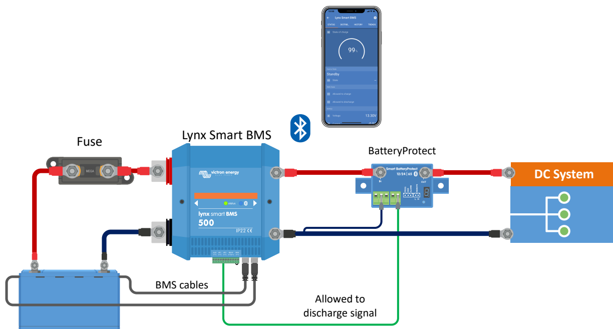
Système avec un Lynx Smart BMS sans autres modules Lynx.
