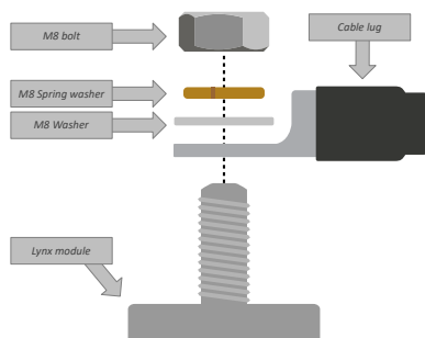
Figure 3. Séquence correcte pour le montage des fils CC.
