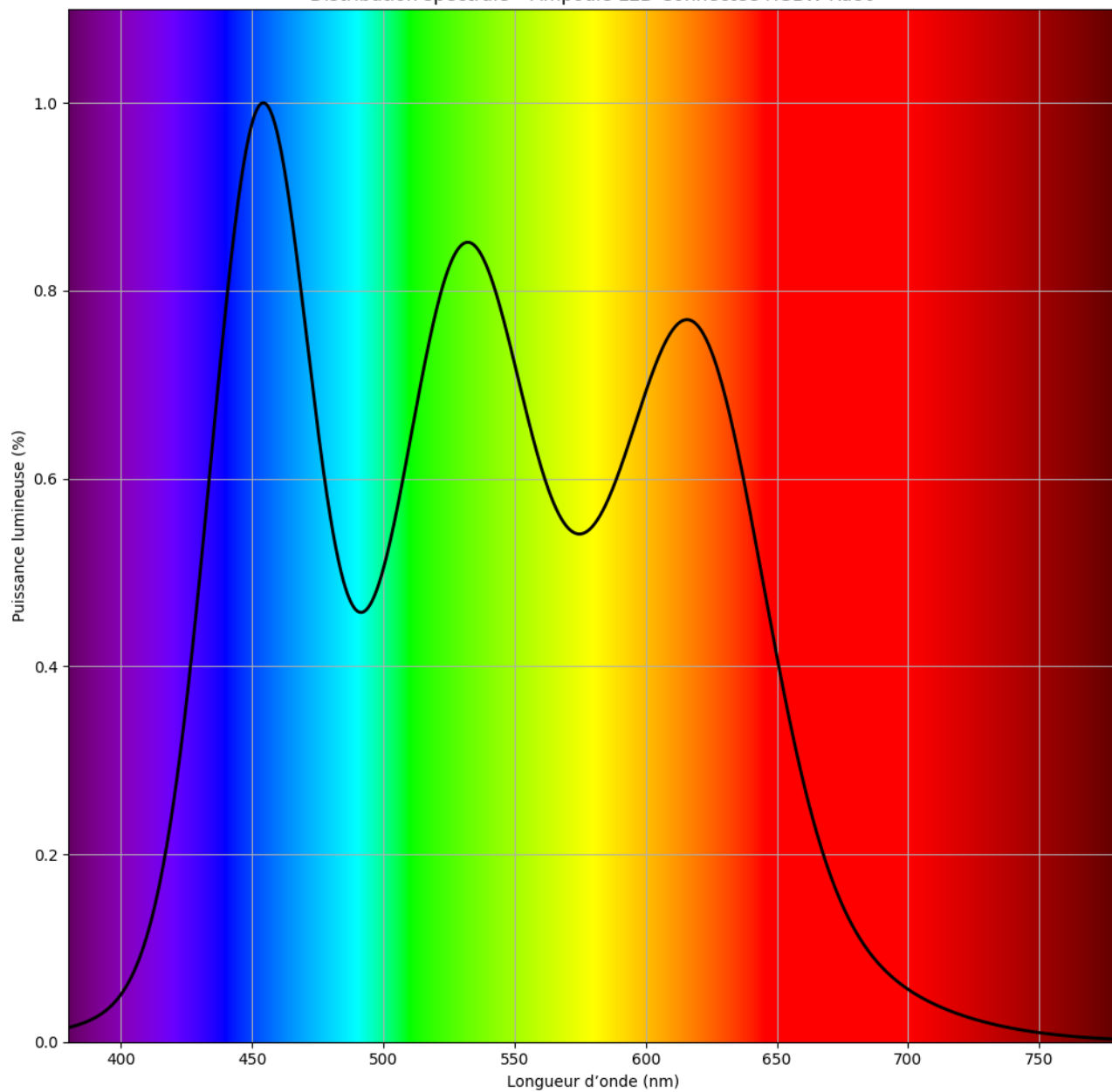
Distribution spectrale - Ampoule LED Connectée RGBW Ra80
