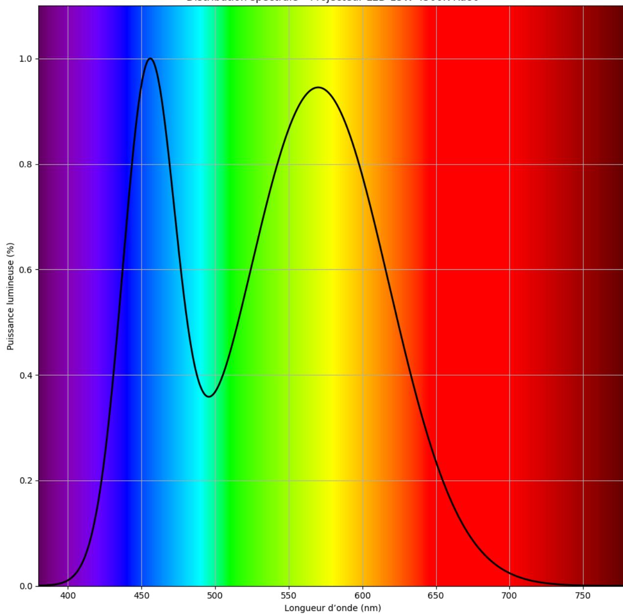
Distribution spectrale - Projecteur LED 15W 4500K Ra80
