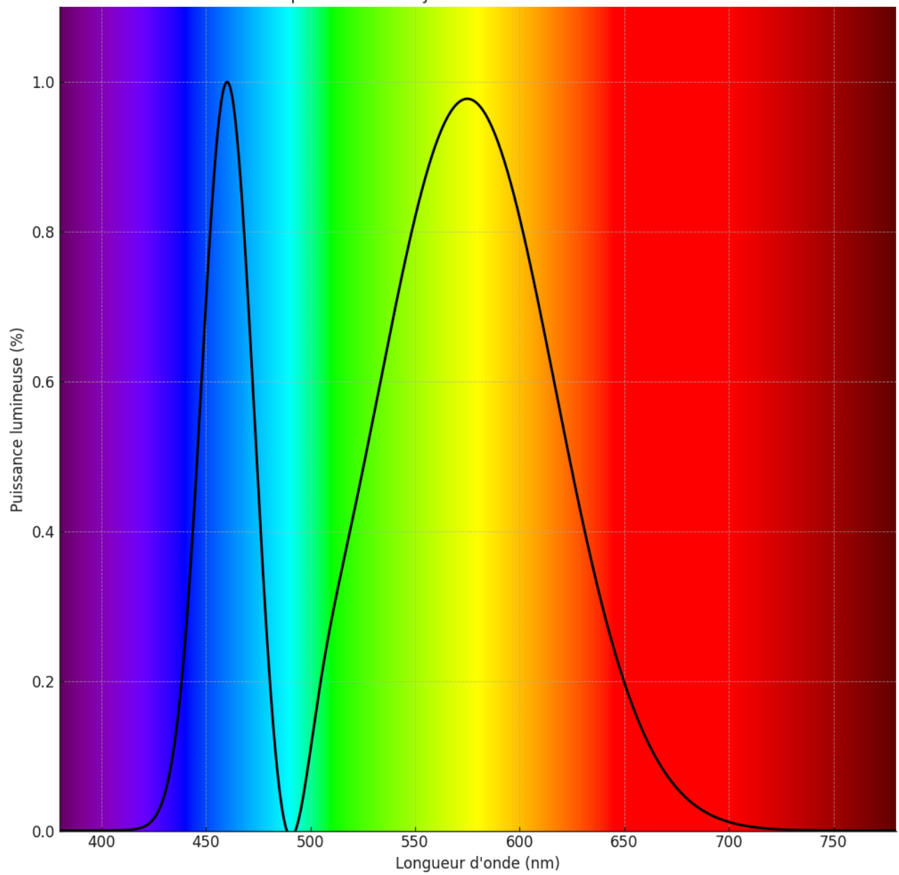
Distribution spectrale - Projecteur LED sur Rail 12W 4200K RA80
