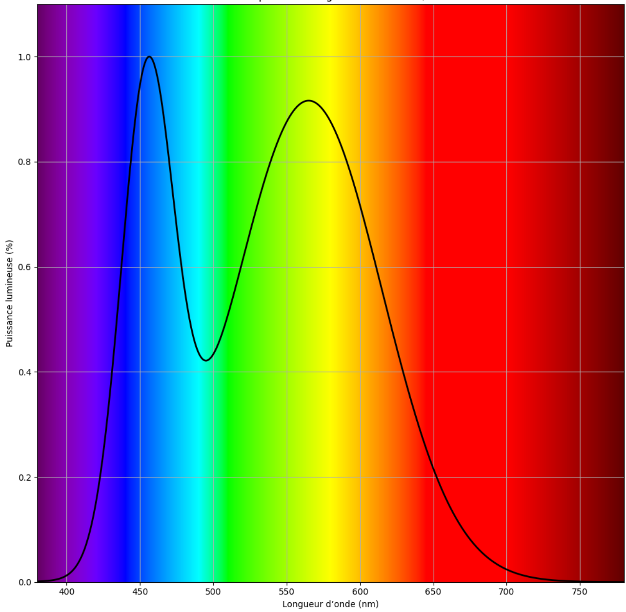
Distribution spectrale - Réglette LED 30cm 1,5W Ra80
