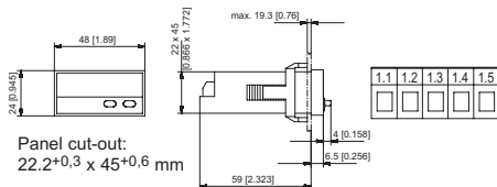
Front bezel
