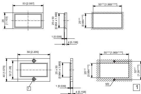
Front bezel
