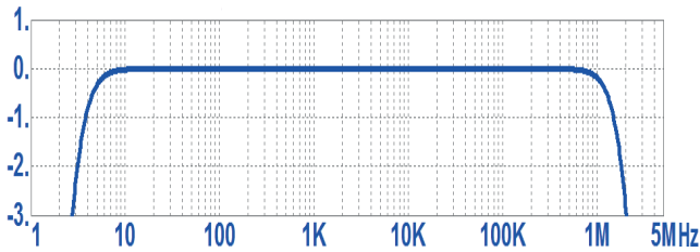
Amplitudenfehler in dB
