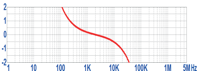
Phasenfehler in Grad
