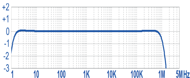
Erreur d'amplitude en dB
