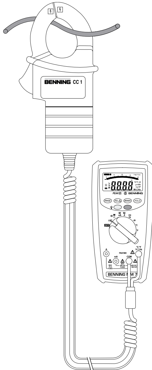
Bild 2: Wechselstrommessung Fig. 2: AC current measurement Fig. 2: Mesure de courant alternatif Fig. 2: Medición de corriente alterna obr. 2: Měření střídavého proudu
