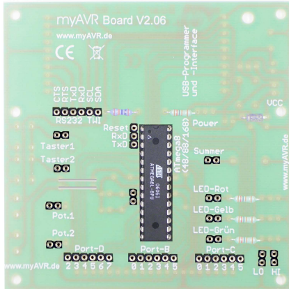
IC-Sockel und Buchsenleisten IC-socket and connector pins
