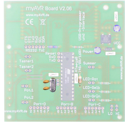
Kondensatoren und Quarz capacitors and quartz
