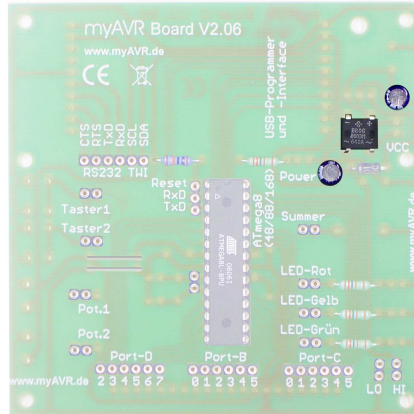
ELKOs: Polarität beachten capacitors: watch polarity
