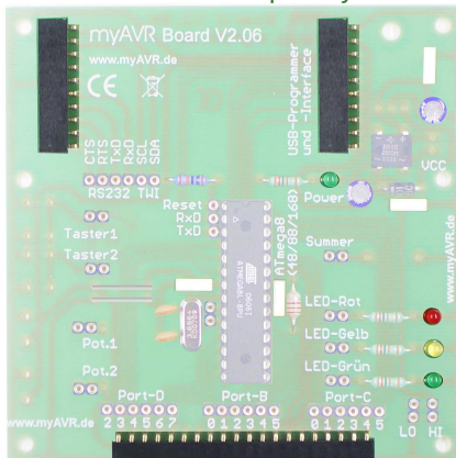
LEDs: Polarität beachten LEDs: watch polarity
