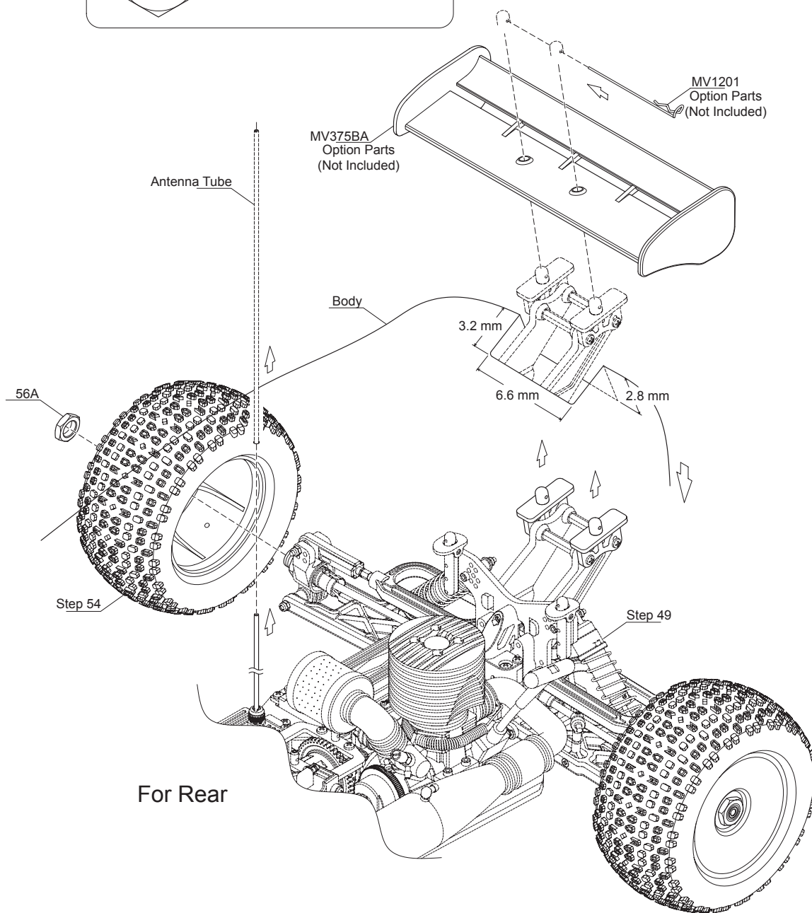
56A -- Wheel Nut 17 mm -- 2
