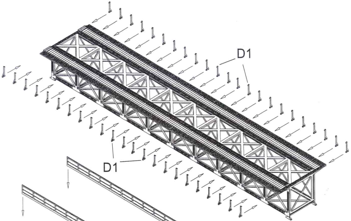
Schritt 7 Step 7
