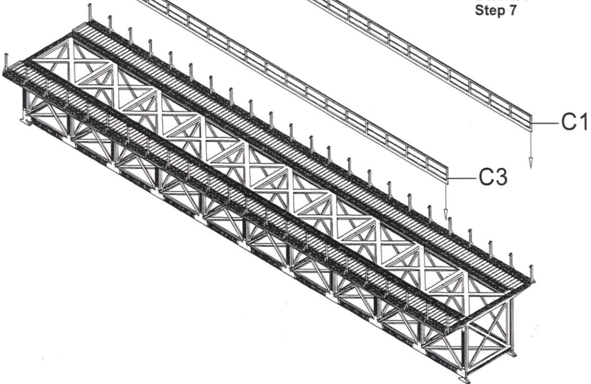
Schritt 8 Step 8
