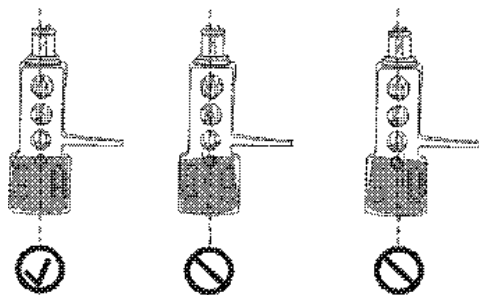
Abb. 9: Einstellen des Azimut
