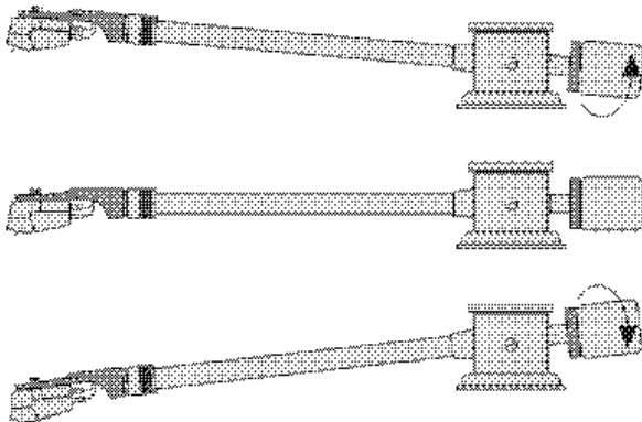
Abb. 4: Tonarm ausbalancieren
