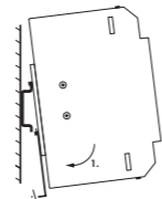
Abb. 2a: Montage
