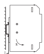
Abb. 2b: Demontage
