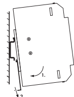
Abb. 2a: Montage
