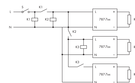
Abb. 3: Parallelschaltung von Netzgeräten
