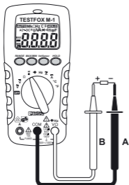
Bild 8: Durchgangsprüfung mit Summer Fig. 8: Continuity testing with buzzer Fig. 8: Contrôle de continuité avec ronfleur Fig. 8: Control de continuidad con vibrador obr. 8: Zkoušku obvodu figur 8: Gennemgangstest med brummer σχήμα 8: Έλεγχος συνέχειας με βομβητή 8. ábra: Folytonosság vizsgálat zűmmögövel ill. 8: Prova di continuità con cicalino Fig. 8: Doorgangstest met akoestisch signaal Rys. 8: Sprawdzenie ciągłości obwodu рис. 8: Проверка целостности цепи Resim 8: Sesli uyarıcı ile süreklilik ölçümü
