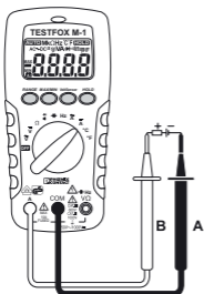
Bild 4: Gleichstrommessung Fig. 4: DC current measurement Fig. 4: Mesure de courant continu Fig. 4: Medición de corriente continua obr. 4: Měření stejnosměrného proudu figur 4: Jævnstrømsmåling σχήμα 4: Μέτρηση συνεχούς ρεύματος 4. ábra: Egyenáram mérés ill. 4: Misura corrente continua Fig. 4: Meten van gelijkstroom Rys.4: Pomiar prądu stałego рис. 4: Измерение величины постоянного тока Resim 4: Doğru Akım Ölçümü
