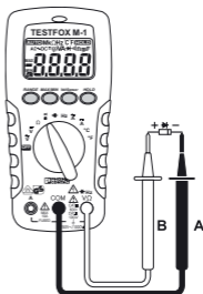
Bild 7: Diodenprüfung Fig. 7: Diode testing Fig. 7: Contrôle de diodes Fig. 7: Verificación de diodos obr. 7: test diod figur 7: Diodelest σχήμα 7: Έλεγχος διόδου 7. ábra: Dióda vizsgálat ill. 7: Prova diodi Fig. 7: Diod-test Rys. 7: Pomiar diody рис. 7: Проверка диодов Resim 7: Diyot Kontrolü
