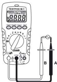
Bild 5: Wechselstrommessung Fig. 5: AC current measurement Fig. 5: Mesure de courant alternatif Fig. 5: Medición de corriente alterna obr. 5: Měření střídavého proudu figur 5: Vekselsstrømsmåling σχήμα 5: Μέτρηση εναλλασσόμενου ρεύματος 5. ábra: Váltakozó áram mérés ill. 5: Misura corrente alternata Fig. 5: Meten van wisselstroom Rys.5: Pomiar prądu przemiennego рис. 5: Измерение величины переменного тока Resim 5: Alternatif Akım Ölçümü
