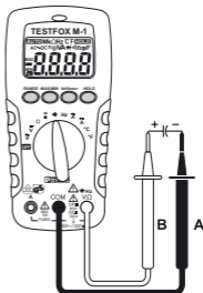
TESTFOX M-1 Bild 9: Kapazitätsmessung Fig. 9: Capacity testing Fig. 9: Mesure de capacité Fig. 9: Medición de capacidad obr. 9: Měření capacity figur 9: Kapacitansmåling σχήμα 9: Μέτρηση χωρητικότητας 9. ábra: Kapacitás mérés ill. 9: Misura di capacità Fig. 9: Capaciteitsmeting Rys. 9: Pomiar pojemności рис. 9: Измерение емкости Resim 9: Karasite Ölçümü
