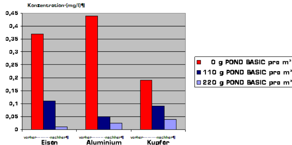
Entfernung von Eisen (Fe), Aluminium (Al) und Kupfer (Cu) aus dem Teichwasser durch FIAP premiumcare POND BASIC
