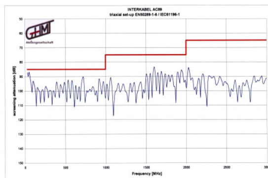
Schirmdämpfung (AC 89):
