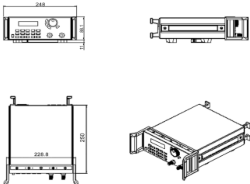
Bild 1-1 Abmessungen des elektronischen, programmierbaren SSL Last-KONSTANTERS, Serie 32 EL
