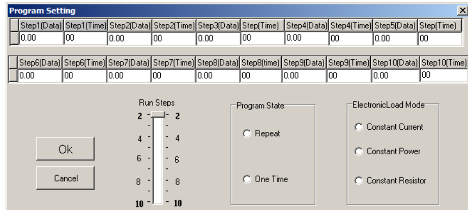
Bild 2-15 Programmfenster
