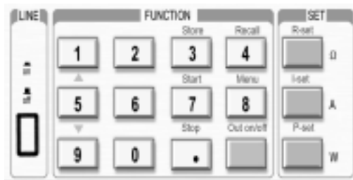
Bild 1-4 Tastenfeld des elektronischen SSL KONSTANTERS, Serie 32 EL
