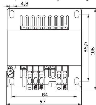
Höhe über alles / overall depth: 106mm
