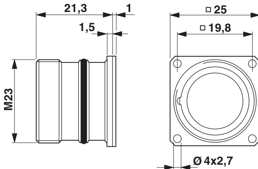
Maßzeichnung
